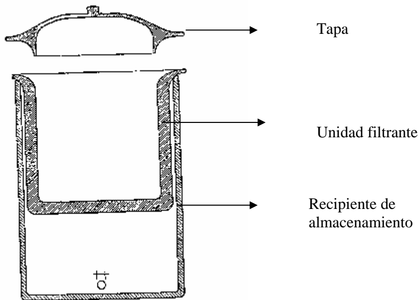
Figura 1. Partes del filtro de cerámica Fuente: Potters for Peace, 2000.
