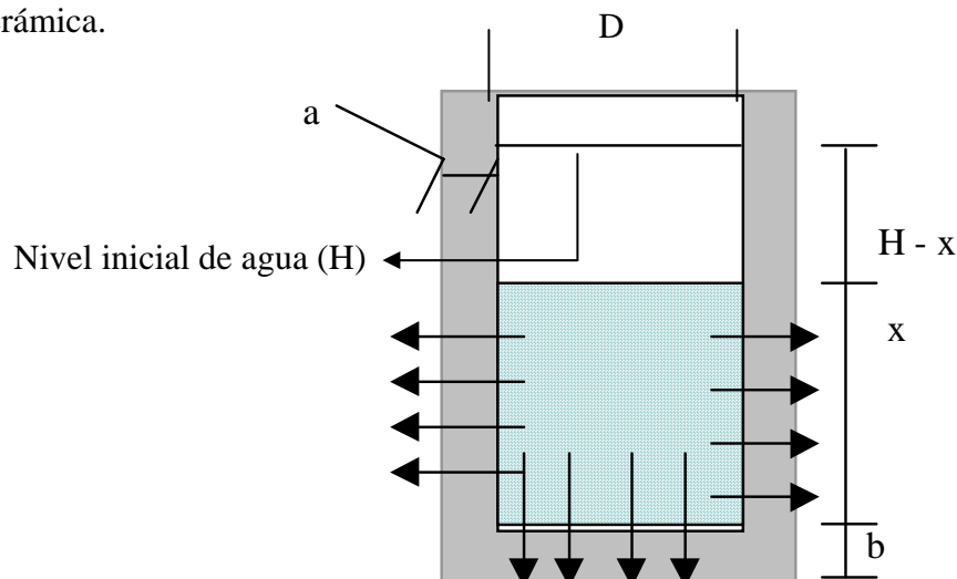
Figura. 2 Corte transversal del filtro de cerámica Fuente: Eriksen, 2000
